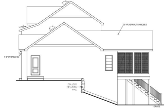
RIGHT ELEVATION
